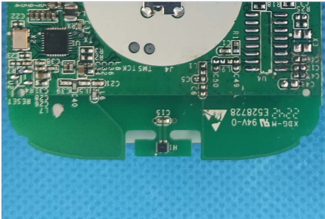
Antenna
