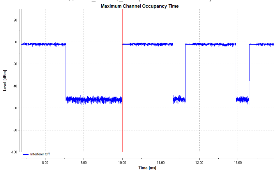
802.11b_Chain 0_2412(COT&Min Idel Period)
